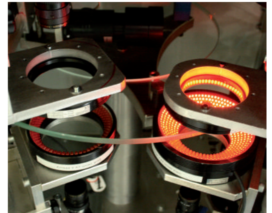
1초에 최대 10개 부품을 검사하는 100% 자동화된 광학 검사 장비
