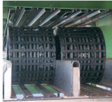
석탄 하역용 쉽 로더(ship loader)에 사용된 확장 링크를 포함한 E4 시리즈.
