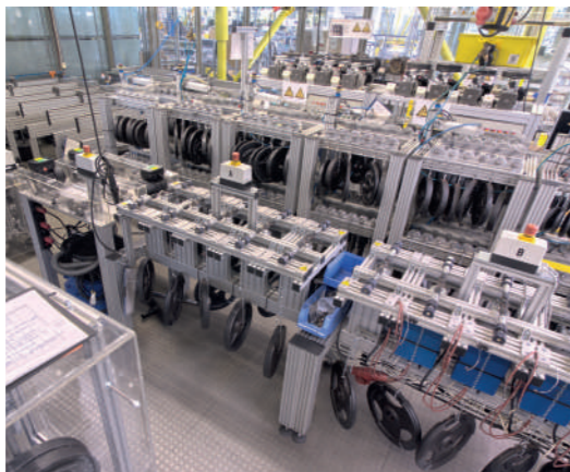
dry테크 테스트 장비
