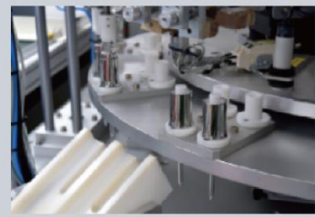
드롭퍼 조립기
